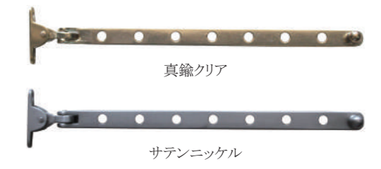
スイング窓固定金物 七つ目真鍮調整アーム (スイング窓1カ所につき1個必要)
